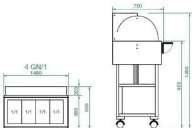
Dimensões do buffet móvel Design Plus 4xGn1/1 com rolltop
